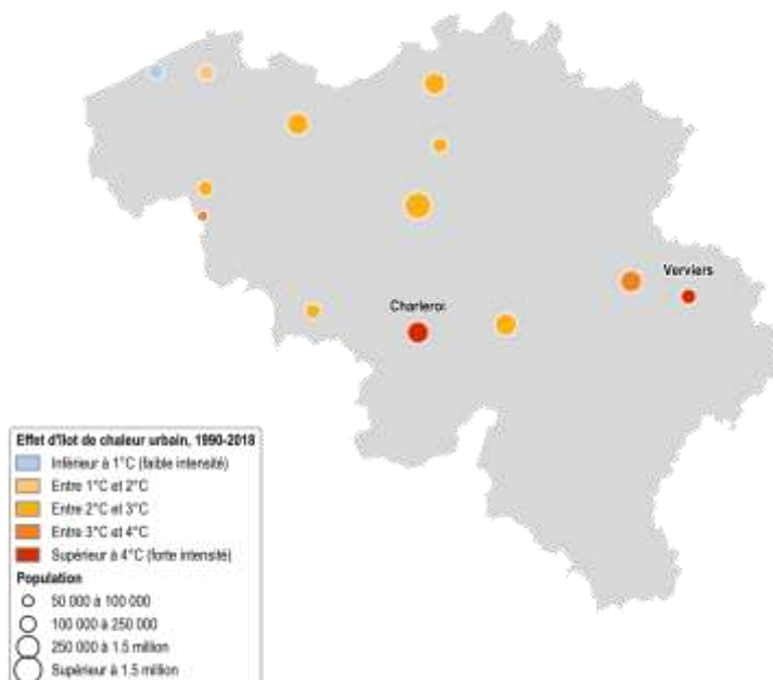
Figure 20: L'effet d'îlot de chaleur urbain, 2021
